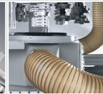
Gesteuerte Absaugung – beste Lösung am Markt
