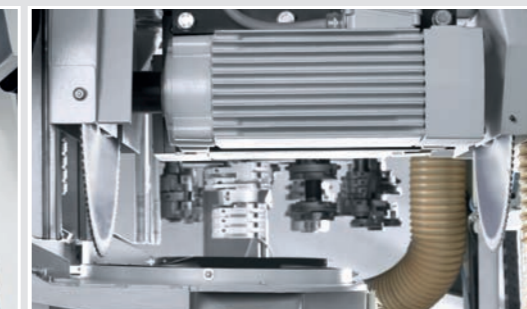
Sägeaggregat zum Ablängen in der Maschine
