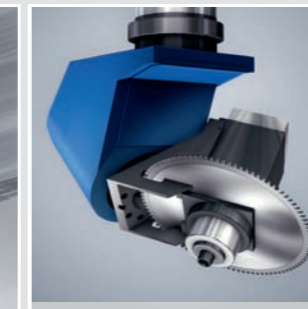
5-Achs-Kopf zum Sägen, Bohren und Profilieren
